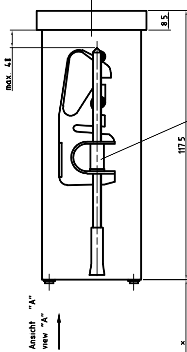
Befestigungsspannen zur Montage abnehmbar clamps for assembly removable
